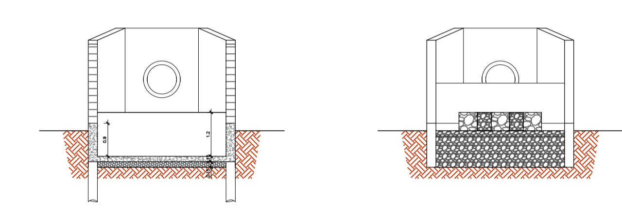
DETALHES DO DISSIPADOR ESCALA 1:100
