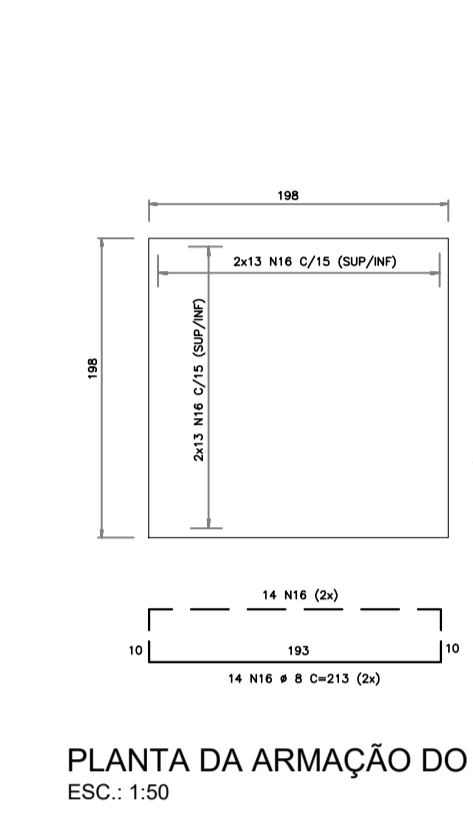
POÇO DE VISITA ESCALA 1:50
