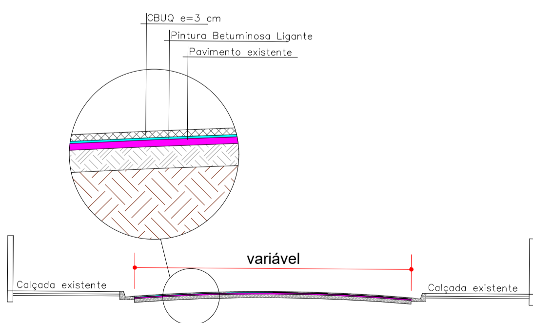
PERFIL TRANSVERSAL GERAL ESCALA 1:100
