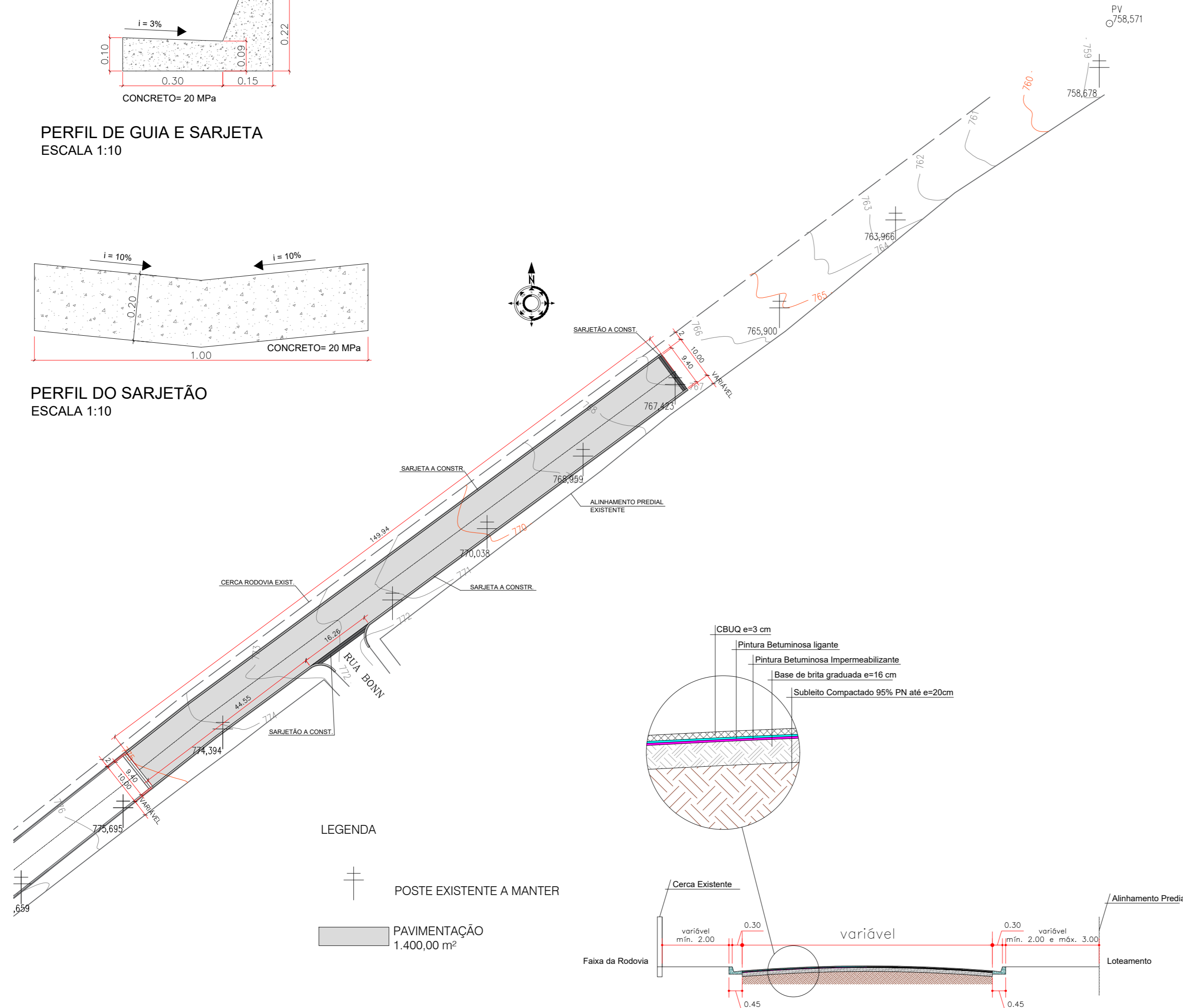
PLANTA BAIXA DE PAVIMENTAÇÃO ESCALA 1:750
