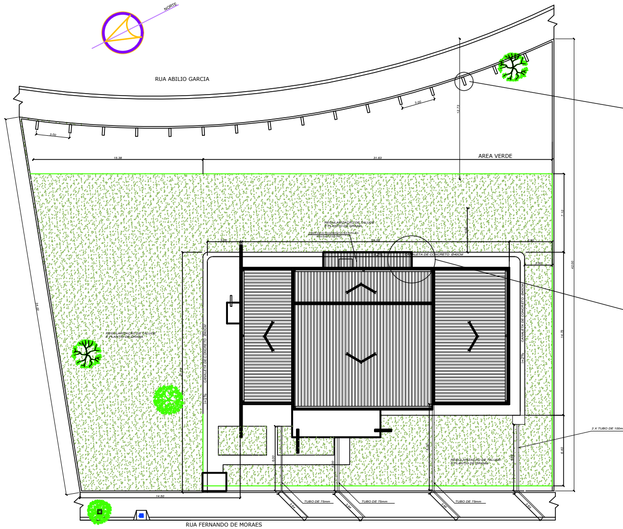
PLANTA DE IMPLANTAÇÃO / COBERTURA ESC. 1:100
