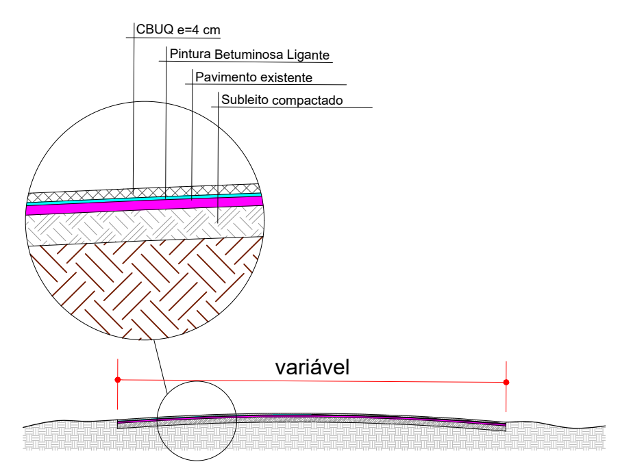
PERFIL TRANSVERSAL GERAL ESCALA 1:100
