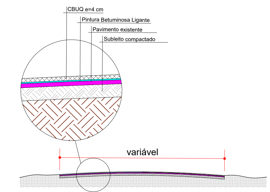
PERFIL TRANSVERSAL GERAL ESCALA 1:100
