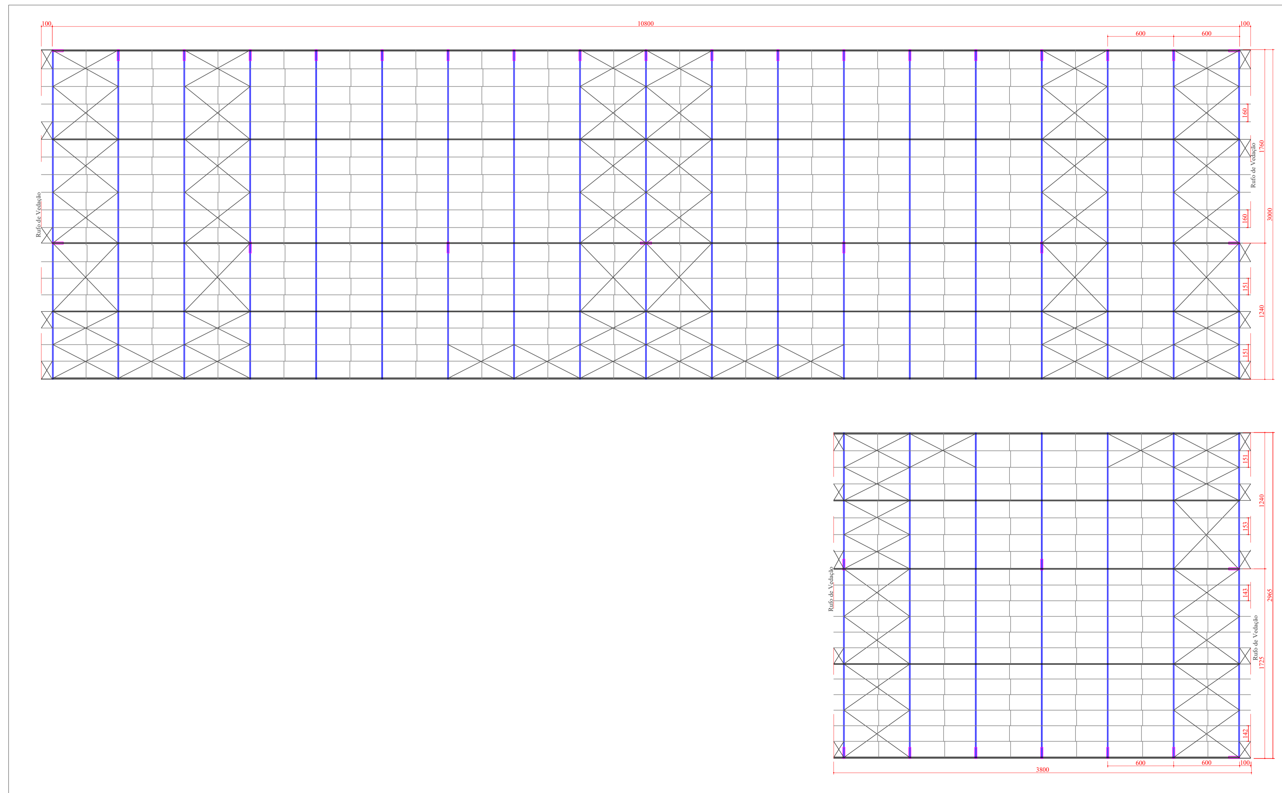
PLANO DE CONTRAVENTAMENTO ESCALA 1:200
