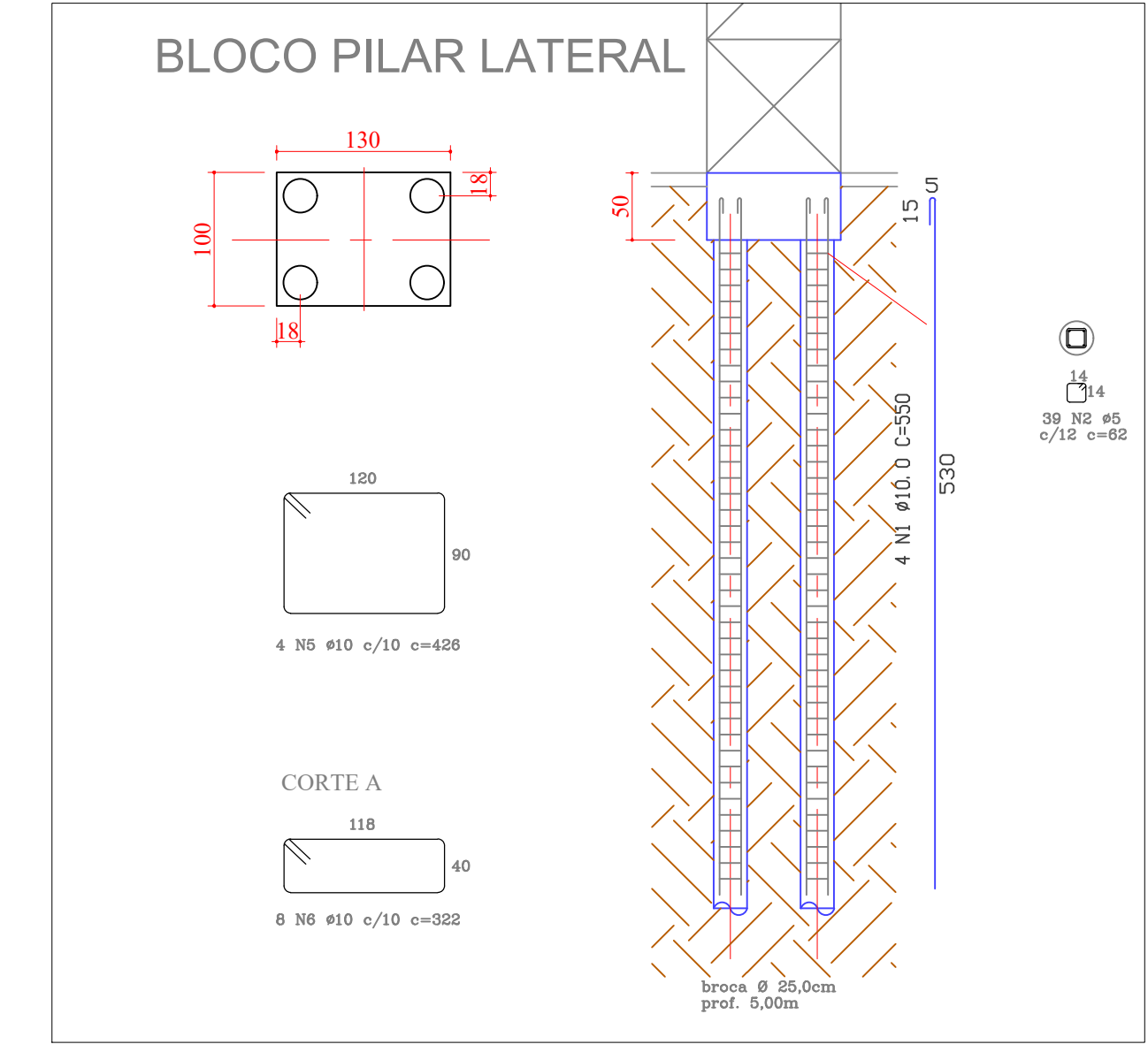
DETALHE FUNDAÇÃO PILARES CENTRAIS E LATERAIS ESCALA 1:50
