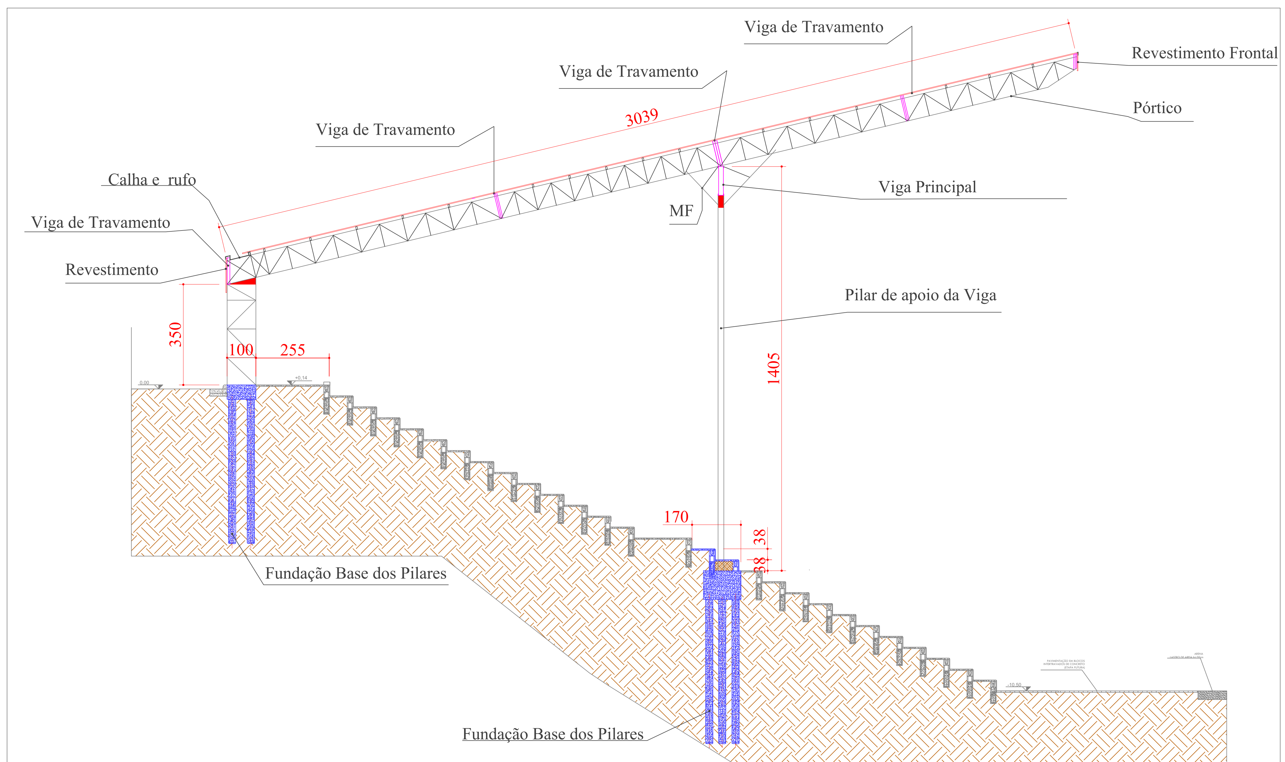
CORTE FF ESCALA 1:75
