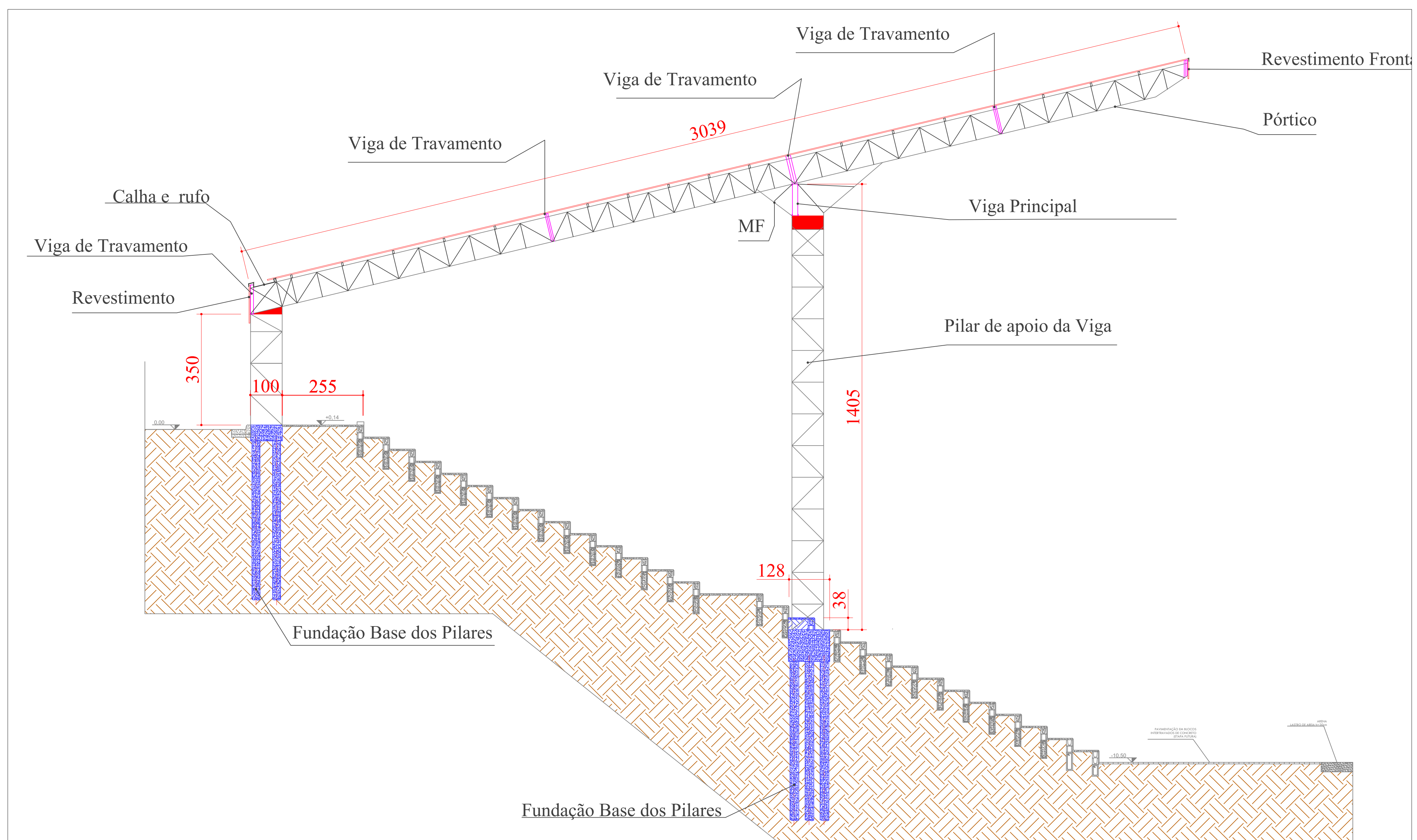
CORTE EE ESCALA 1:75
