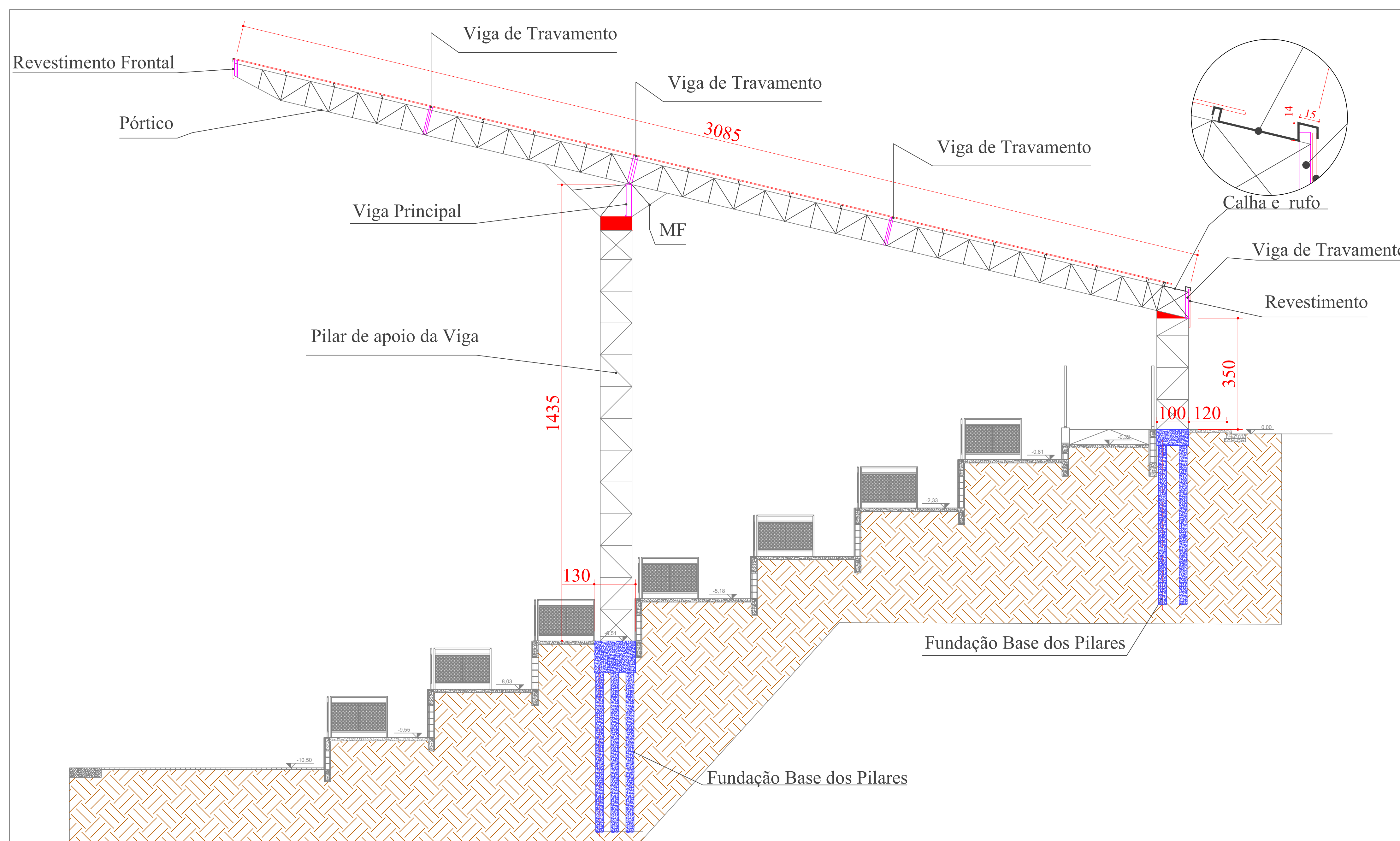
CORTE AA ESCALA 1:75
