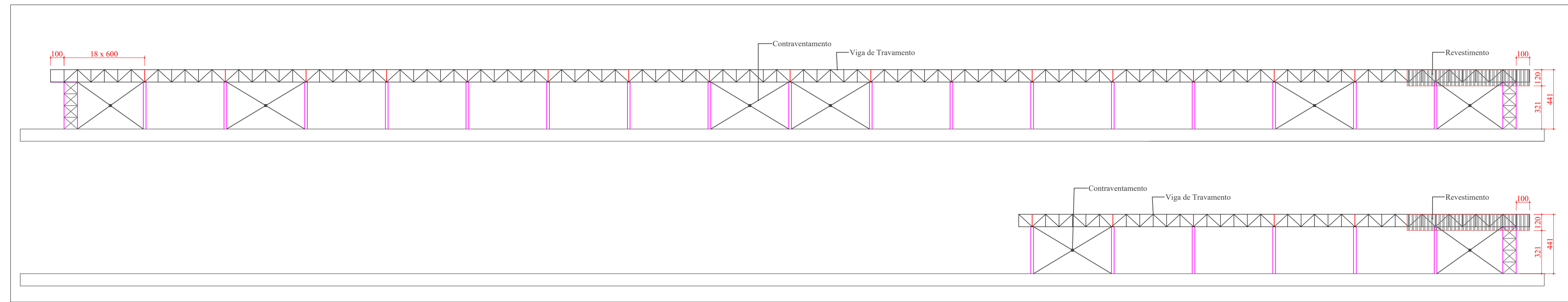
PERFIL LONGITUDINAL ESCALA 1:200
