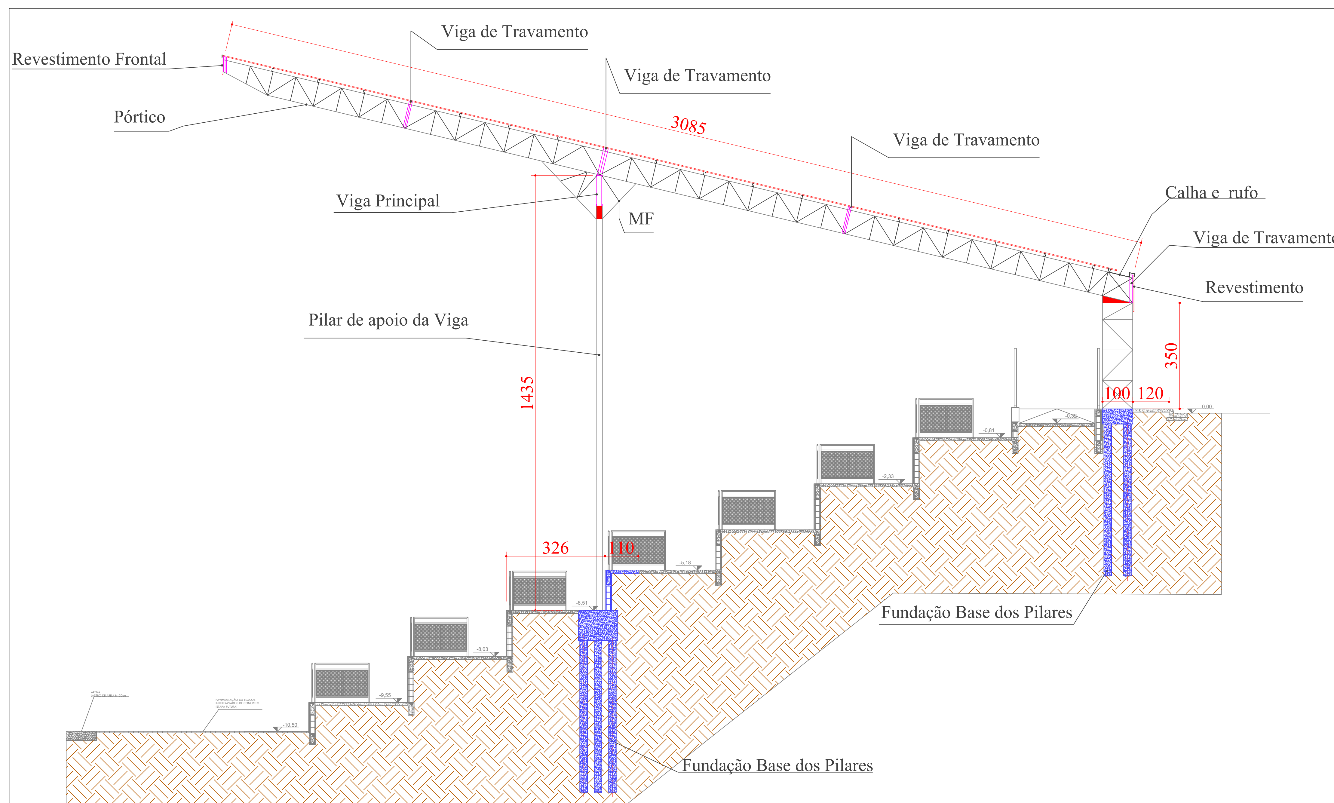
CORTE BB ESCALA 1:75
