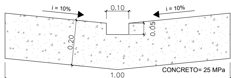
PERFIL DO SARJETÃO L=1,00m ESCALA 1:10
