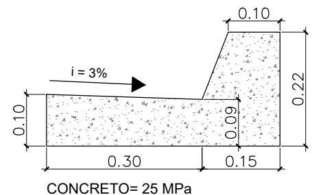
PERFIL DE GUIA E SARJETA EXTRUSADA ESCALA 1:10
