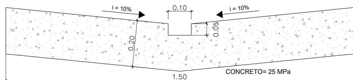
PERFIL DO SARJETÃO L=1,50m ESCALA 1:10
