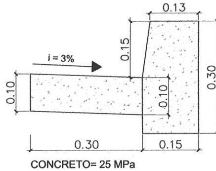
PERFIL DE GUIA PRÉ-MOLDADA E SARJETA MOLDADA "IN LOCO" ESCALA 1:10
