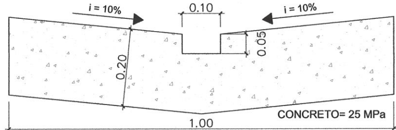
PERFIL DO SARJETÃO L=1,00m ESCALA 1:10
