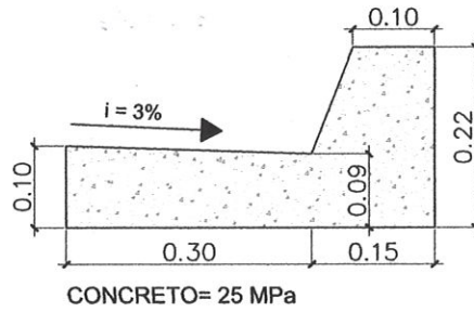
PERFIL DE GUIA E SARJETA EXTRUSADA ESCALA 1:10
