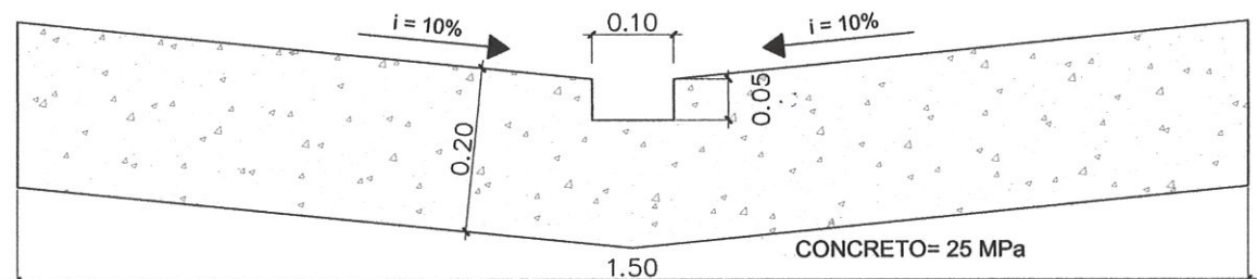
PERFIL DO SARJETÃO L=1,50m ESCALA 1:10
