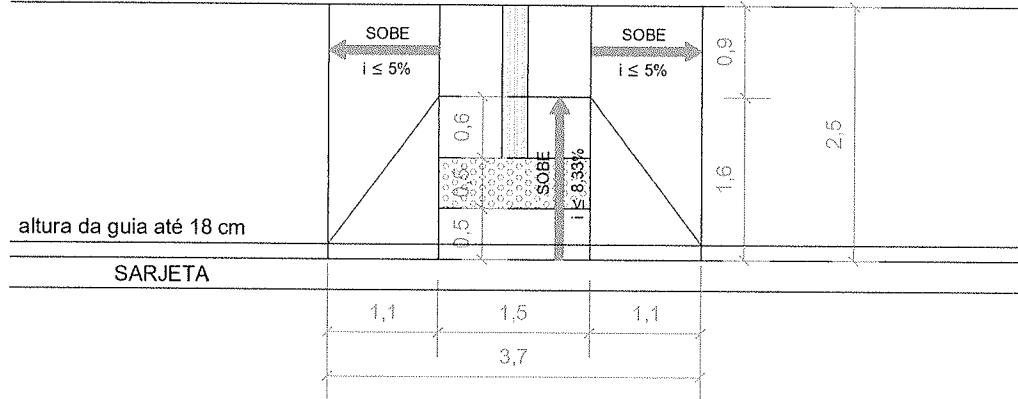
MODELO 03 - REBAIXAMENTO DE CALÇADAS COM RAMPAS COMPLEMENTARES Escala 1:75
