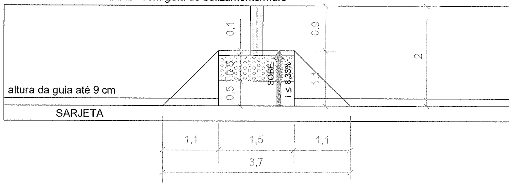
MODELO 02 - REBAIXAMENTO DE CALÇADAS COM PEQUENO DESNÍVEL DE SARJETA Escala 1:75
