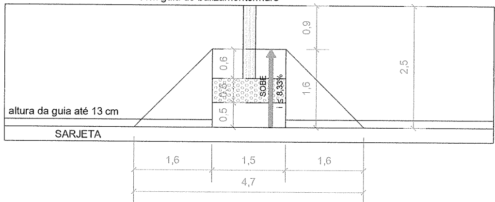
MODELO 04 - REBAIXAMENTO DE CALÇADAS COM PEQUENO DESNÍVEL DE SARJETA Escala 1:75
