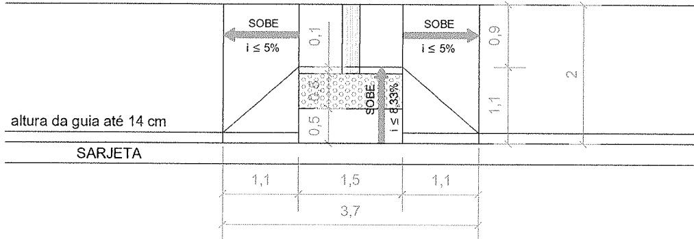
MODELO 01 - REBAIXAMENTO DE CALÇADAS COM RAMPAS COMPLEMENTARES Escala 1:75
