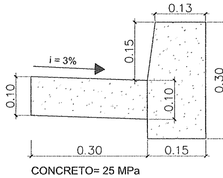
PERFIL DE GUIA PRÉ-MOLDADA E SARJETA MOLDADA "IN LOCO" ESCALA 1:10
