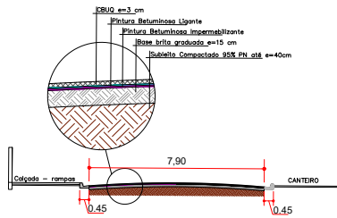
PERFIL TRANSVERSAL GERAL SEM ESCALA
