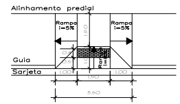
PLANTA-DISPOSITIVO DE ACESSIBILIDADE
