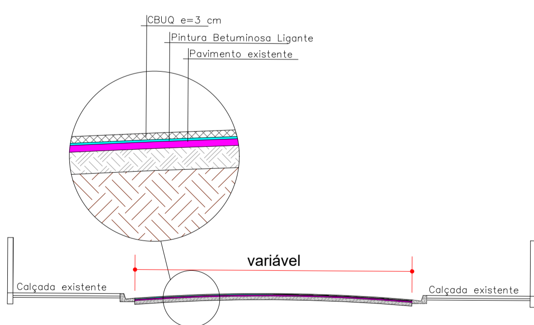
PERFIL TRANSVERSAL GERAL ESCALA 1:100
