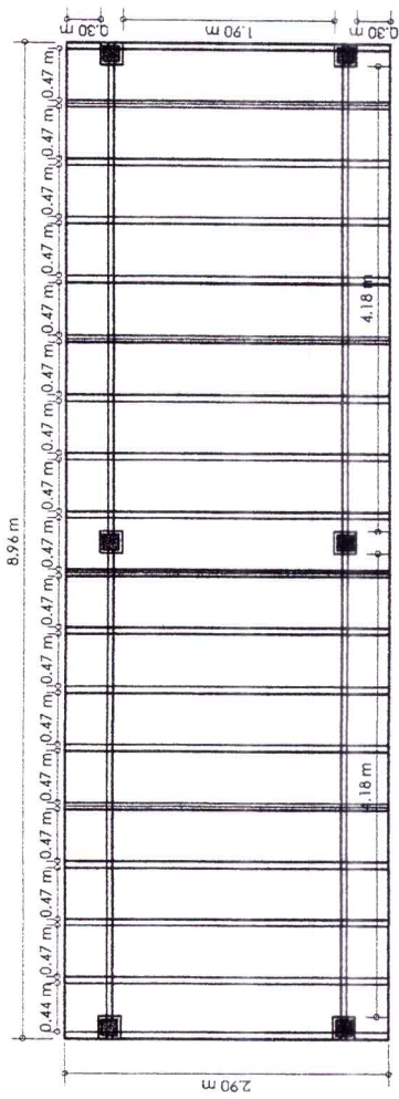
PLANTA - PERGOLADO 02
