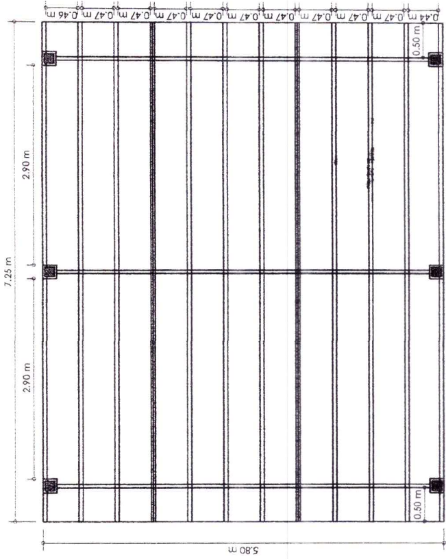
PLANTA - PERGOLADO 01
