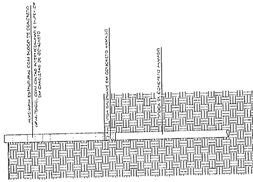
CORTE AA Folha 1/10
